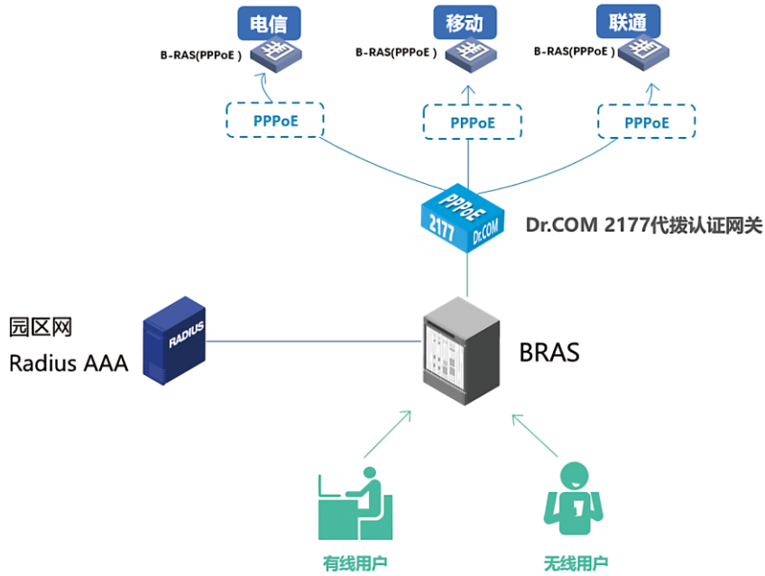
串接单机部署模式
