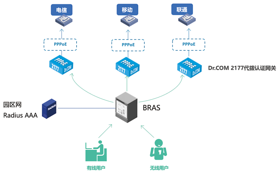
串接多机部署模式
